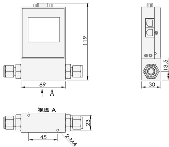
▲ ACU20P-LM 压力计
