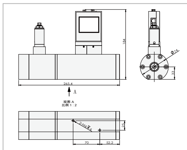
▲ACU20FC-BC 差压式质量流量控制器 (大量程)
