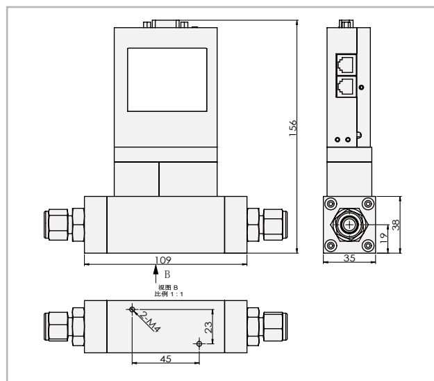
▲ACU20FC-MM 差压式质量流量计 (中量程)
