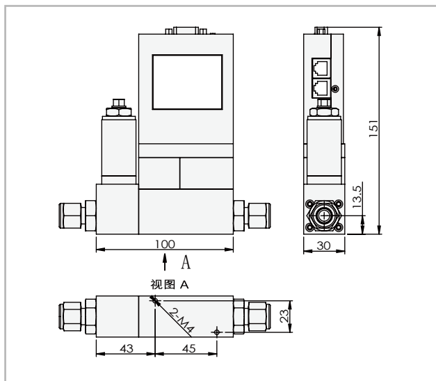
▲ACU20FC-LC 差压式质量流量控制器 (低量程)
