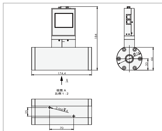
▲ACU20FC-BM 差压式质量流量计 (大量程)
