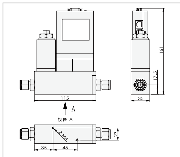
▲ACU20FC-MC 差压式质量流量控制器 (中量程)
