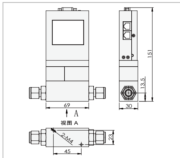
▲ACU20FC-LM 差压式质量流量计 (低量程)
