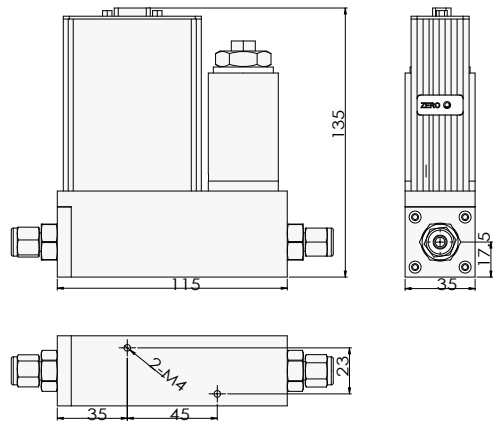
▲ ACU10FA-MC 质量流量控制器
