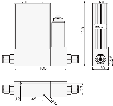
▲ ACU10FA-LC 质量流量控制器
