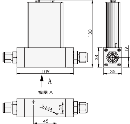
▲ ACU10FA-MM 质量流量计
