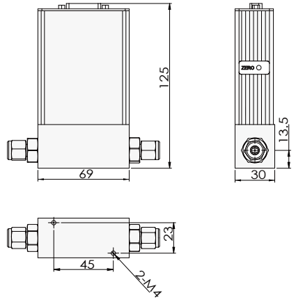
▲ ACU10FA-LM 质量流量计
