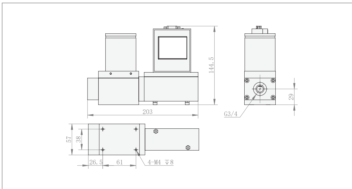
▲ ACU30FCR-BC高精度差压式流量控制器
