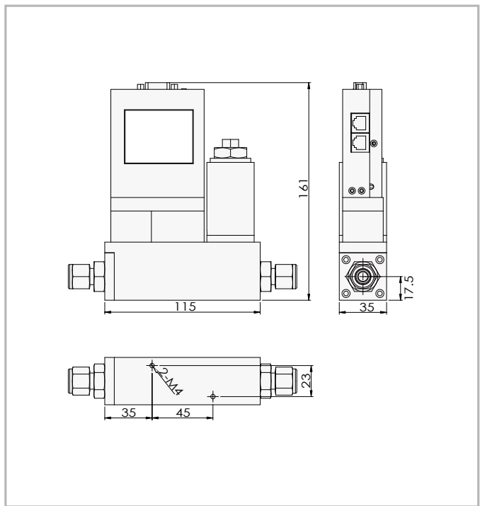
▲ACU20L-MC 液体质量流量控制器 (中量程)
