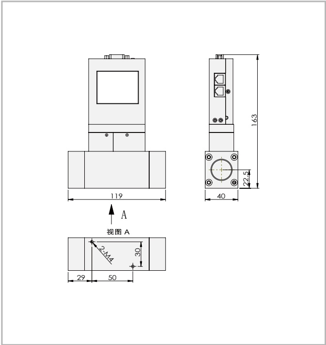
▲ACU20L-BM 液体质量流量计（大量程）
