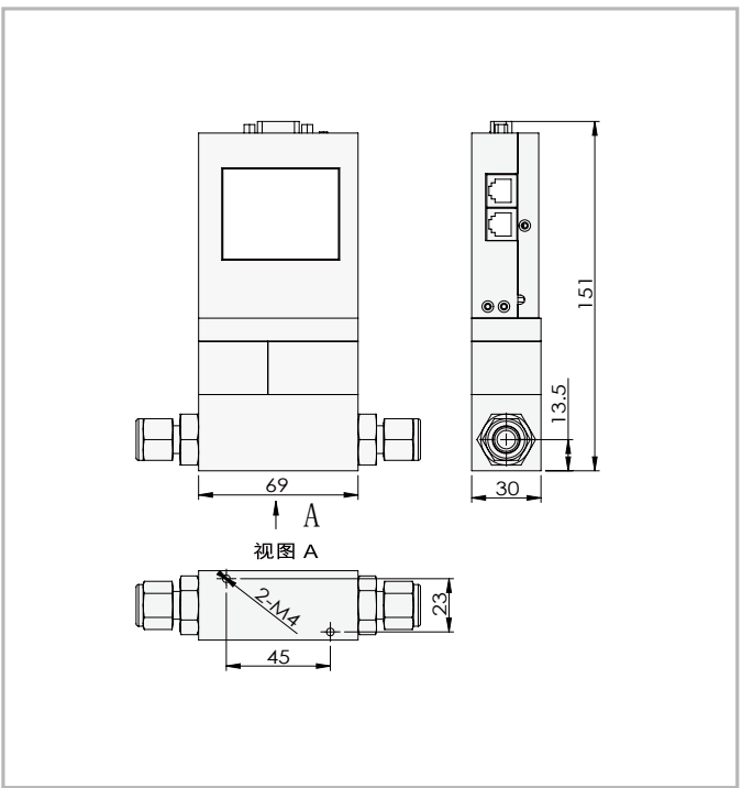
▲ACU20L-LM 液体质量流量计 (低量程)
