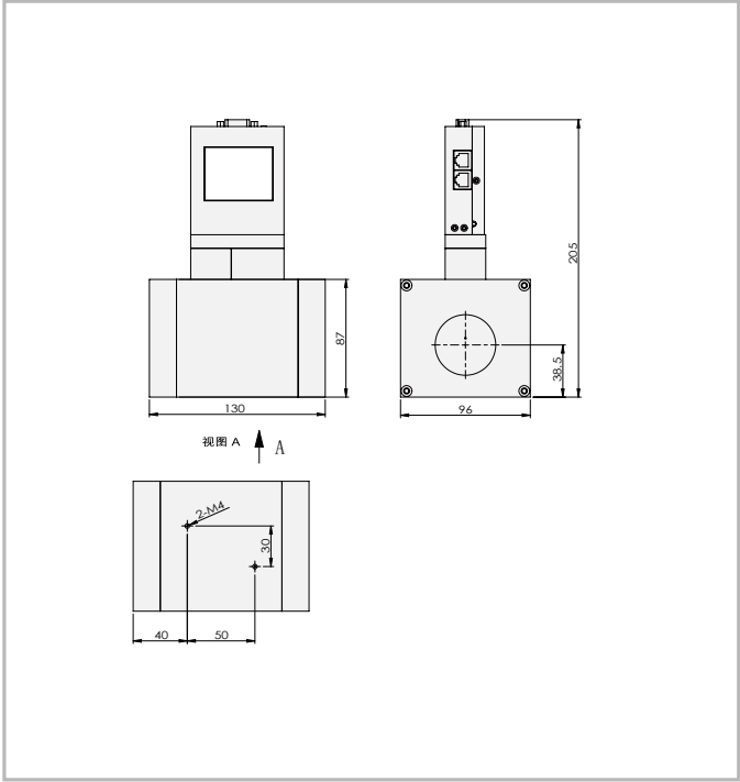
▲ACU20L-HM 液体质量流量计（超大量程）
