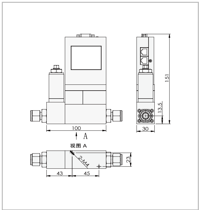
▲ACU20L-LC 液体质量流量控制器 (低量程)
