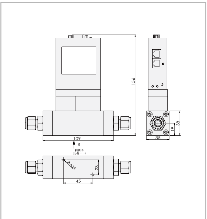
▲ACU20L-MM 液体质量流量计 (中量程)
