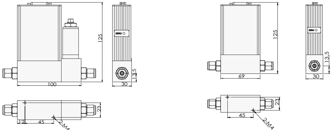
▲ ACU10FA-LC 质量流量控制器
