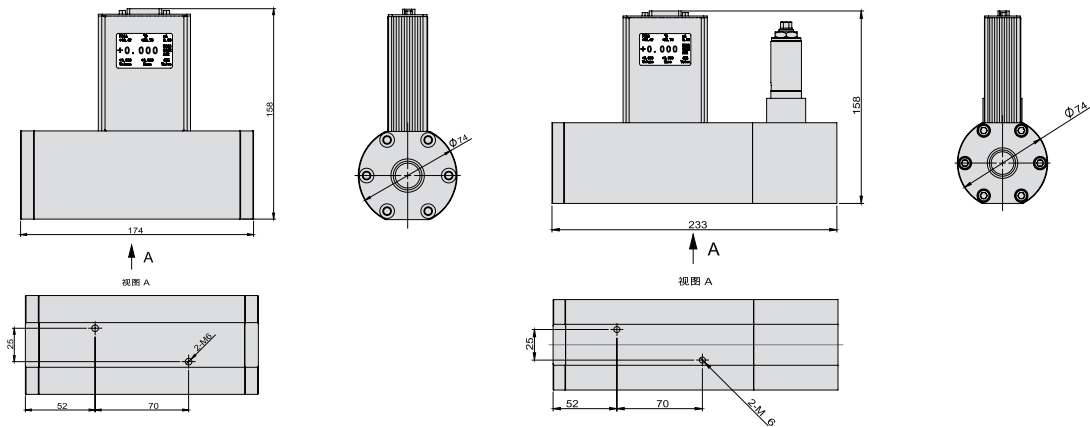
ACU10FD-BM质量流量计
