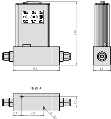
ACU10FD-MM质量流量计
