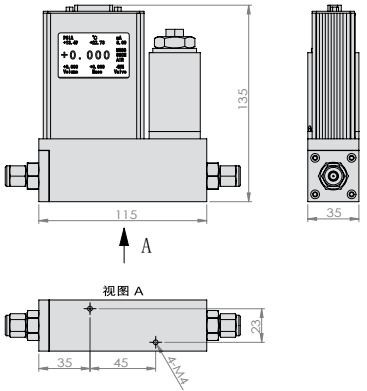
ACU10FD-MC质量流量控制器
