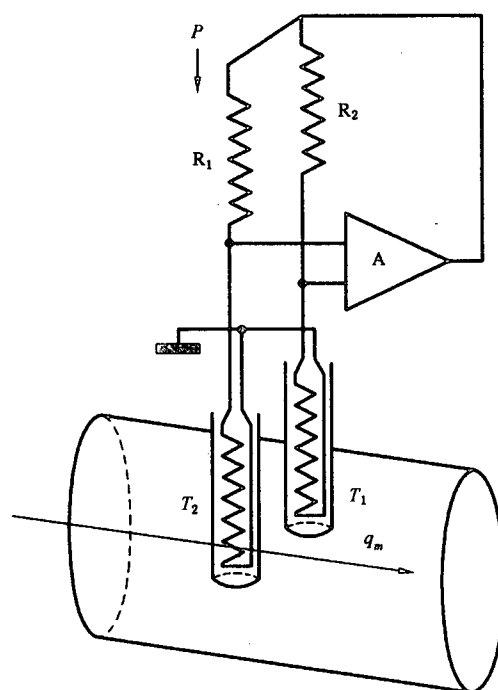
图 4 “恒功率”ITMF 流量计传感器电路简图
