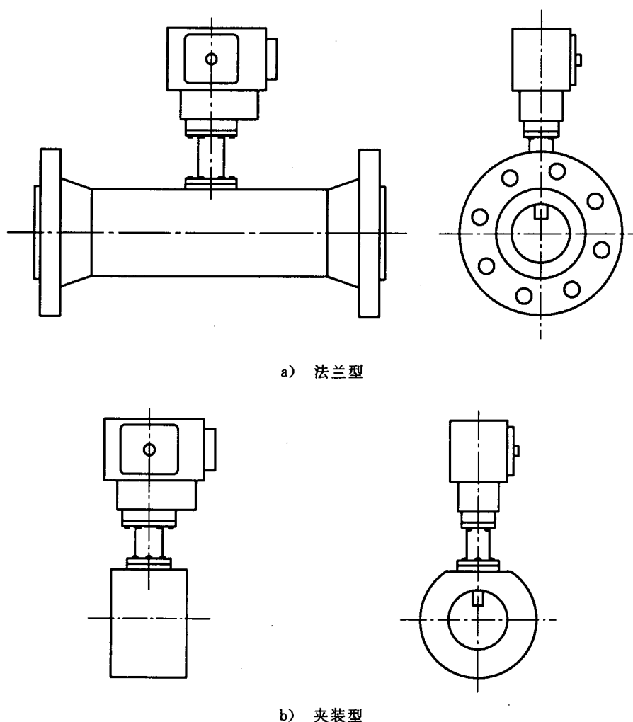
图 6 典型的法兰型和夹装型管道式 ITMF 流量计结构
