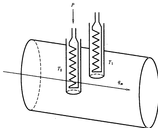
图3 典型的ITMF流量计传感器结构
