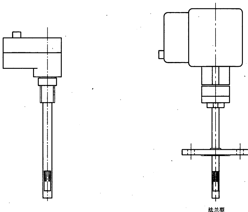
图 7 典型的插入式 ITMF 流量计结构
